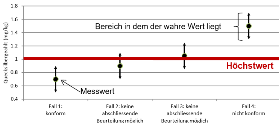
Abbildung 1: Darstellung 4 möglicher Fälle, deren jeweiliger Messwert, die zugehörige Messunsicherheit sowie die daraus abgeleitete Konformitätsbeurteilung.
